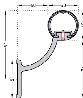
Support plein 60 mm autobloquant en aluminium aspect anodisé argent
