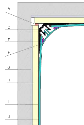
FIN'ANGLE PVC EN MILIEU HUMIDE
