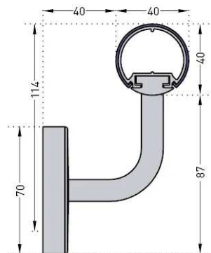
Support col de cygne avec rosace 70 mm autobloquant en inox brossé
