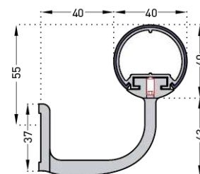
Support galbé 55 mm autobloquant en aluminium aspect anodisé argent
