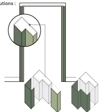
Pliage en U et pliage en L avec joint silicone (huisseries)
